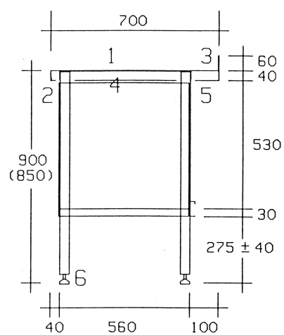
Skeem 1 töölaua mõõdud
